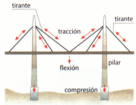
Puente colgante atirantado.
