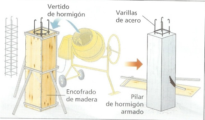
Construcción de un pilar con un encofrado de madera
